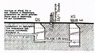
Schnitt Kanal
