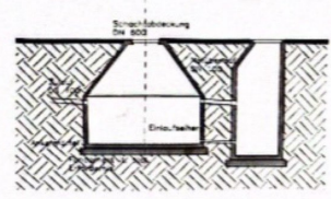
Schnitt Sammelschacht
