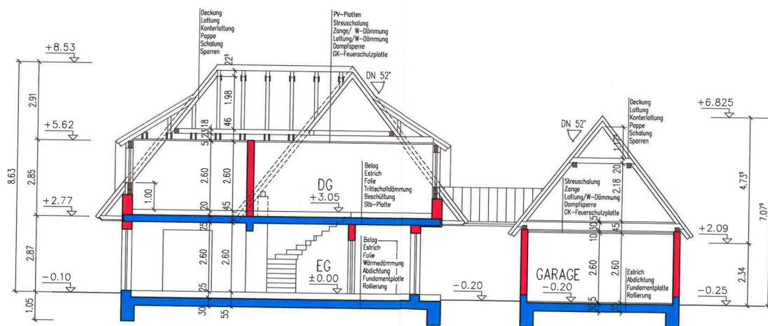
SNITT A-A
