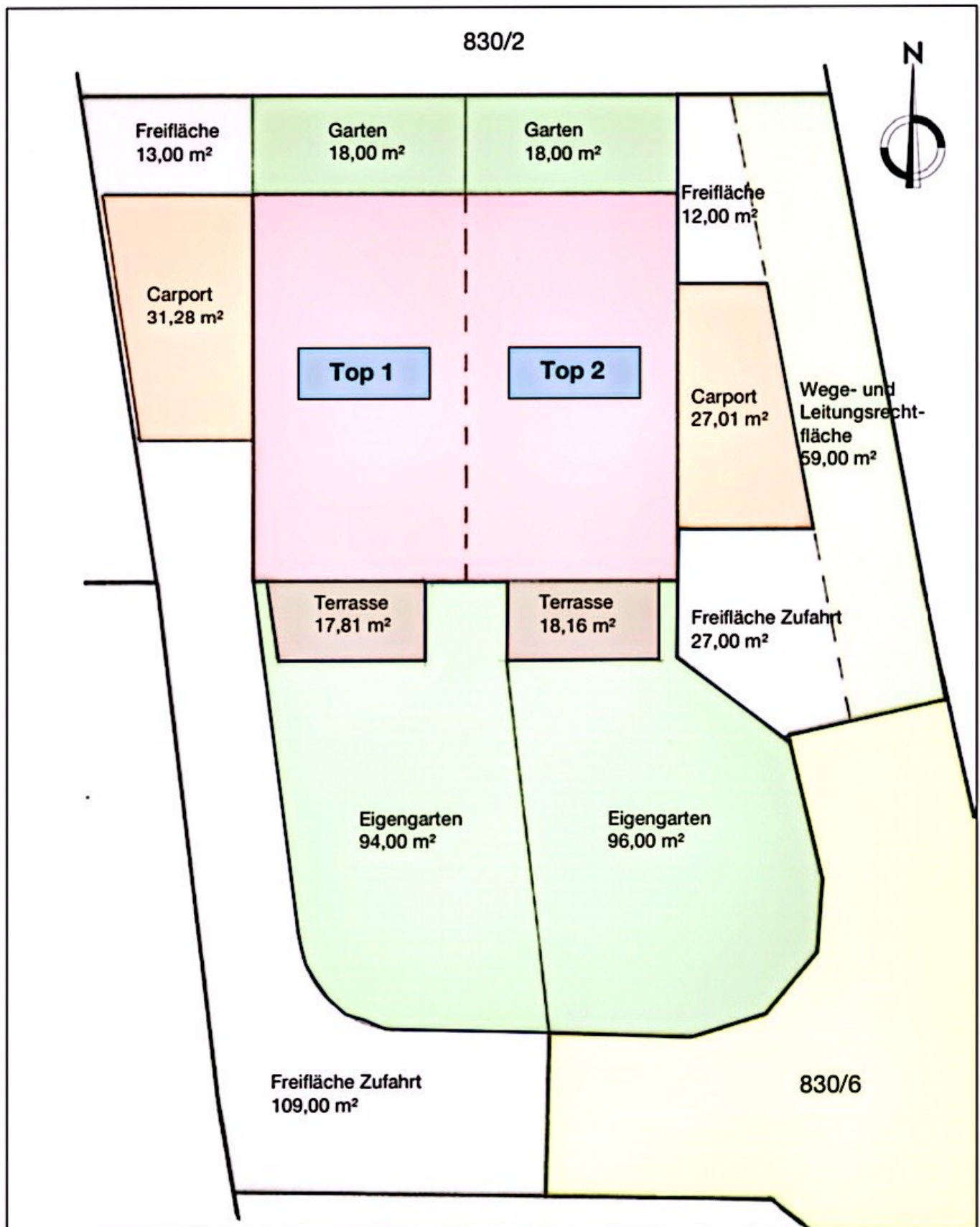
Abbildung 1: Lageplan
