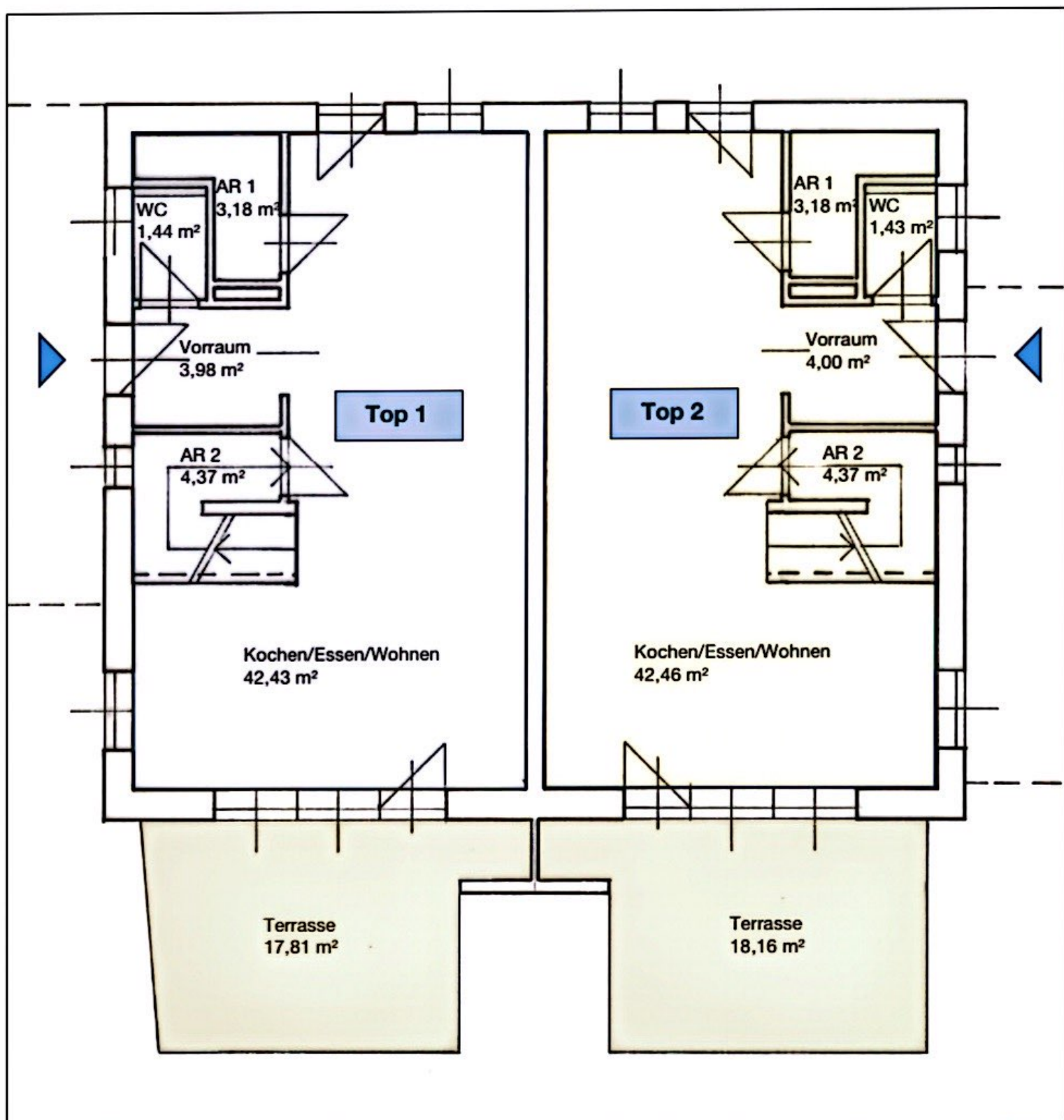
Abbildung 2: Grundriss Erdgeschoss
