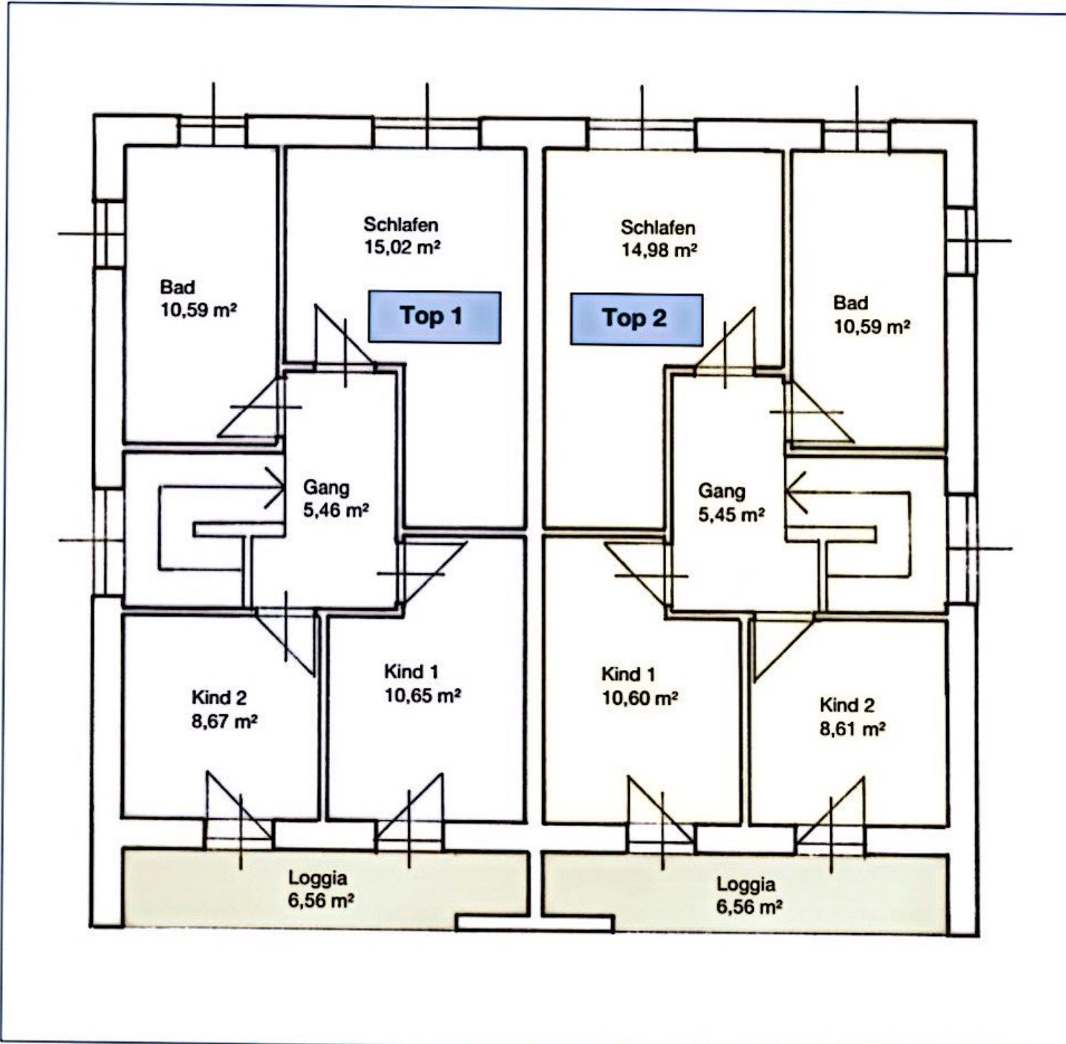
Abbildung 3: Grundriss Obergeschoss
