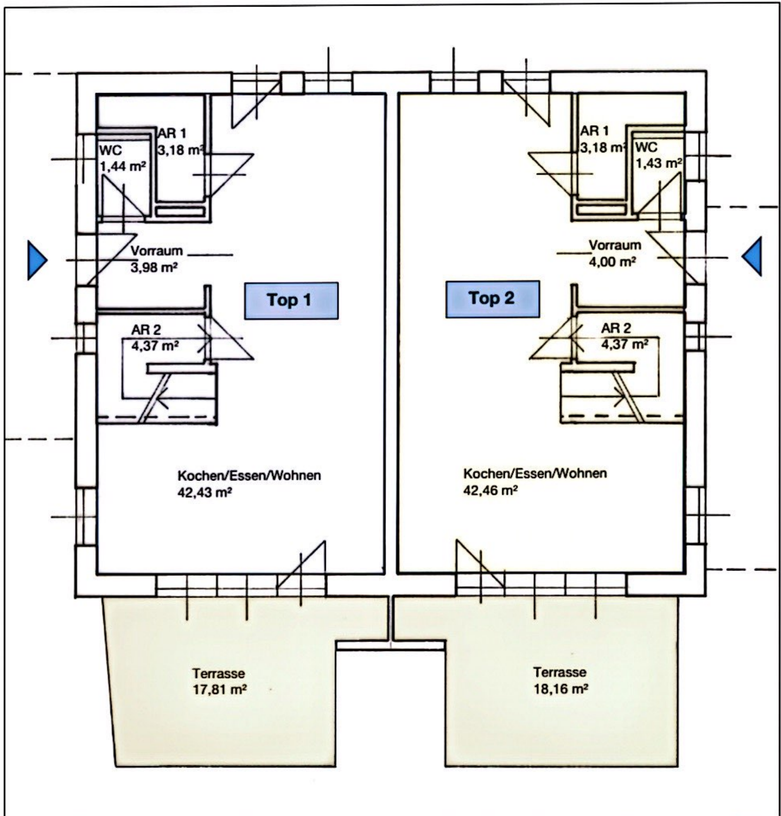
Abbildung 2: Grundriss Erdgeschoss
